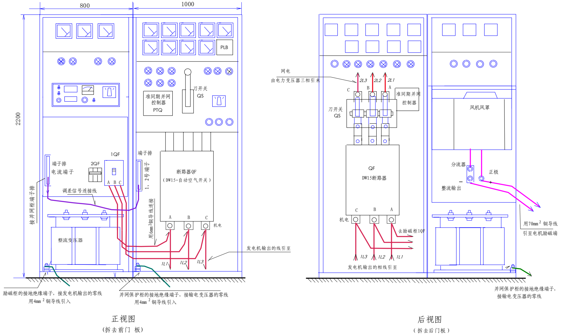
励磁屏与控制屏安装接线示意图
